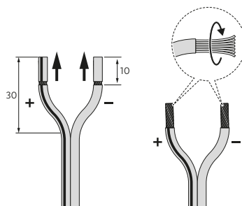
Lautsprecherkabel
