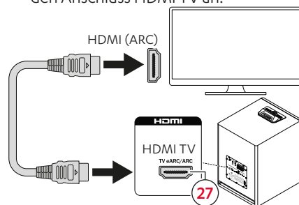
Anschlusskizze HDMI TV
