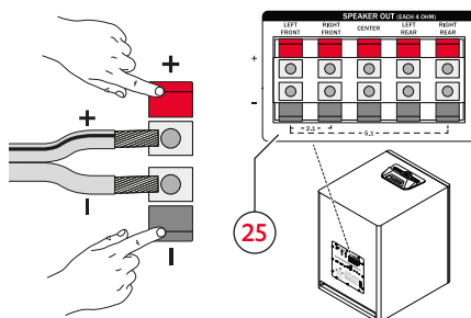
Lautsprecherkabel anschließen
