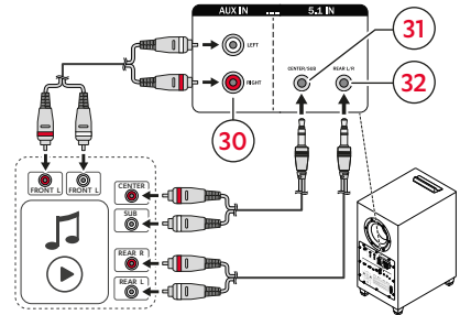
Anschlusskizze 5.1 IN (CENTER/SUB + REAR L/R)
