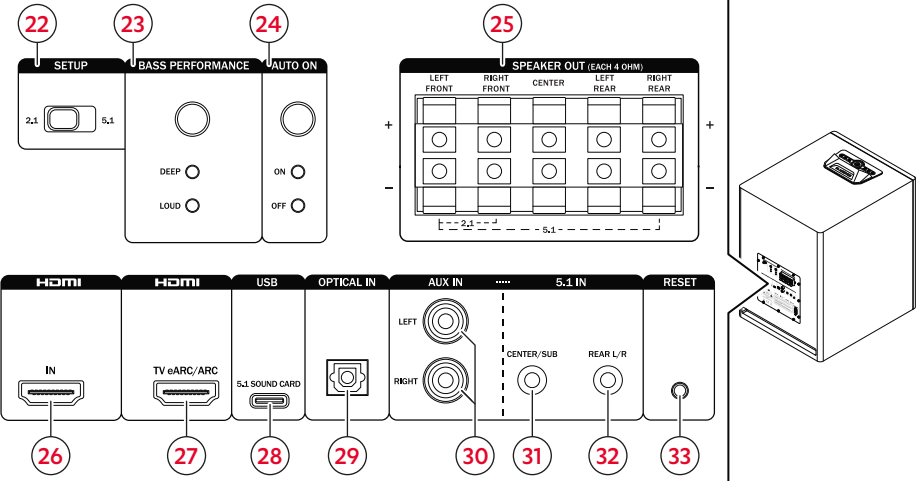
Interrupteurs et ports à l'arrière de l'enceinte
