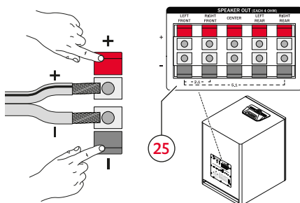
Branchement du câble d'enceinte
