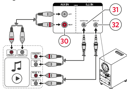
Schéma de connexion 5.1 IN (CENTER/SUB + REAR L/R)
