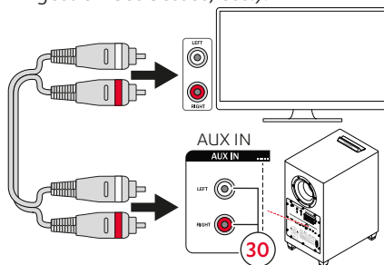
Schéma de connexion AUX IN LEFT/RIGHT
