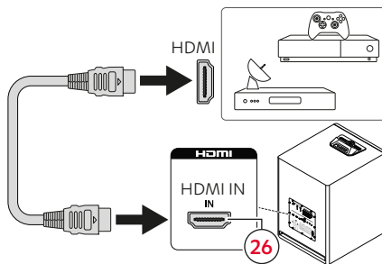
Schéma de connexion HDMI IN
