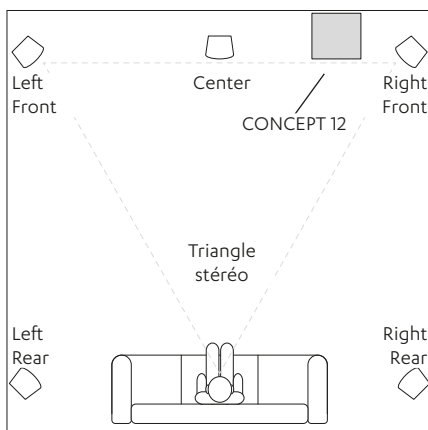
Installation dans l'espace de vie
