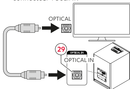
Schéma de connexion OPTICAL IN
