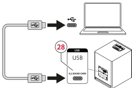
Schéma de connexion PC
