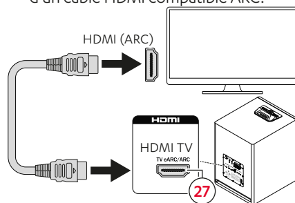
Schéma de connexion HDMI TV
