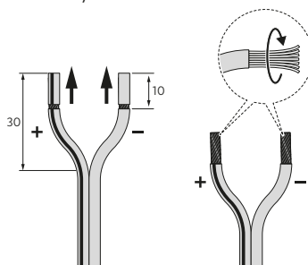
Przygotowanie kabla głośnikowego
