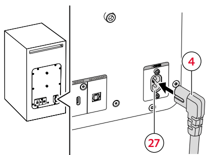
Conexión de alimentación en el altavoz secundario
