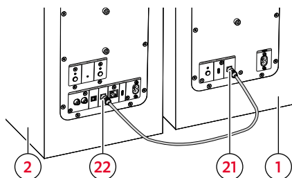
Conexión del cable para altavoz
