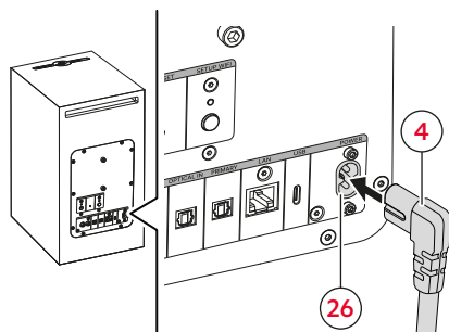
Allacciamento di rete dell'altoparlante primario
