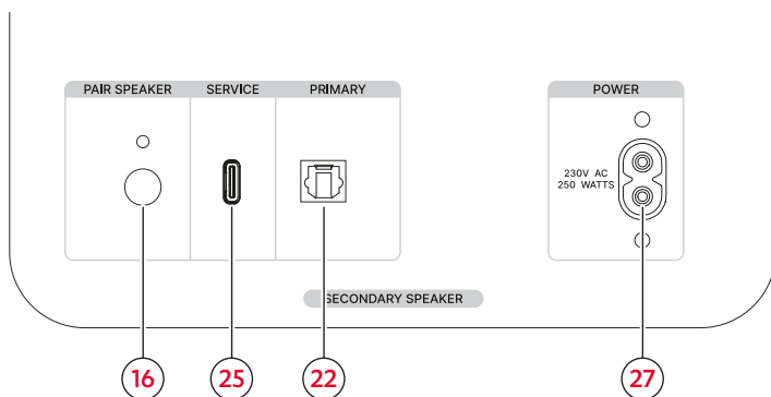
Collegamenti e tasti dell'altoparlante secondario
