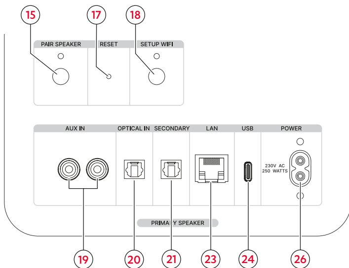
Collegamenti e tasti dell'altoparlante primario
