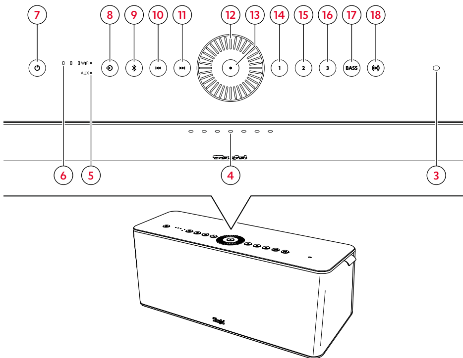
Elementy obsługowe i wskaźniki
