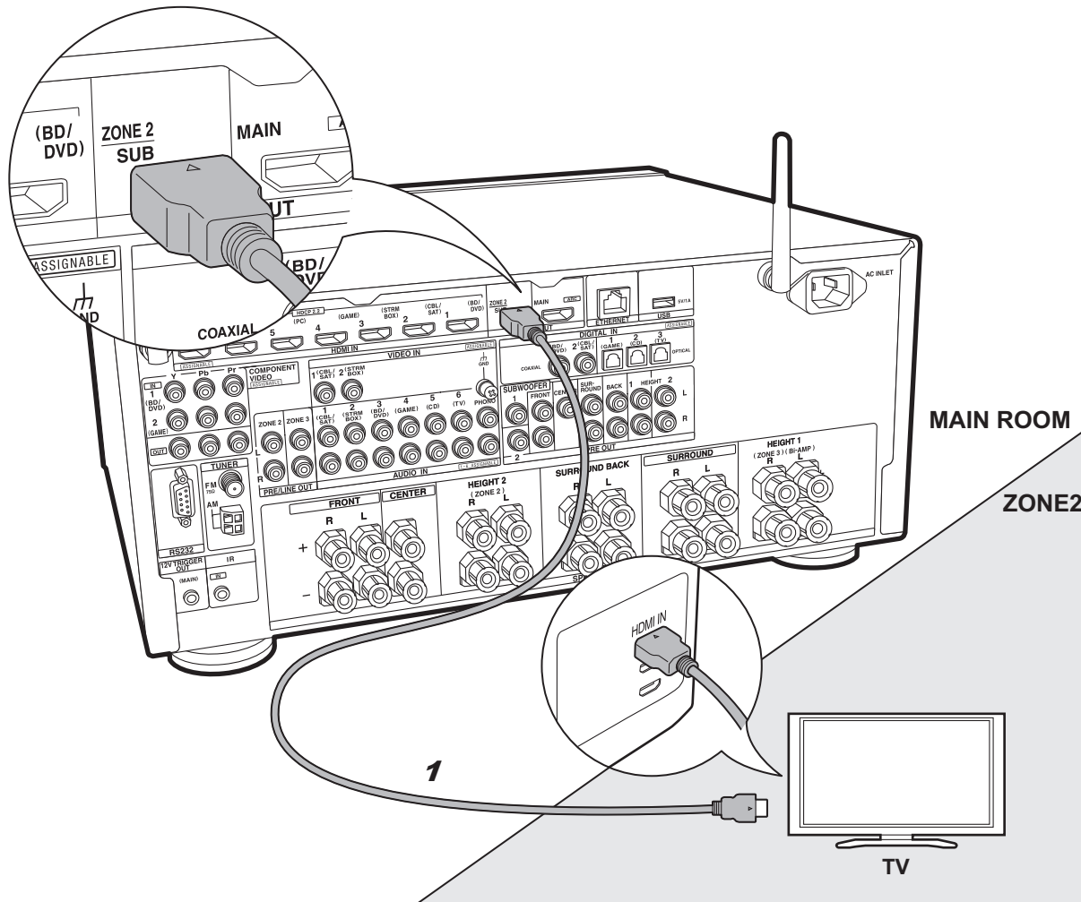
1 HDMI-Kabel
